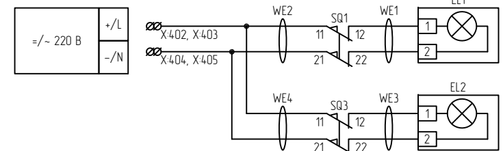
Цепи освещения шкафа
