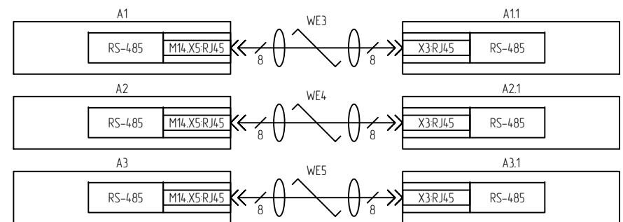
Цепи портов связи терминала
